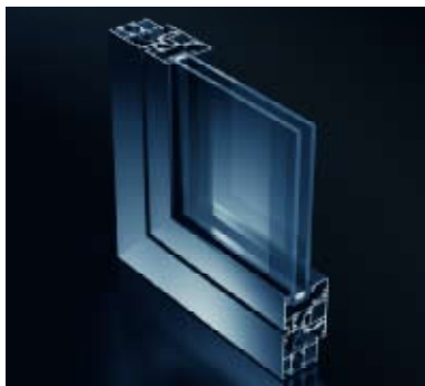
Schüco Window AWS 50
