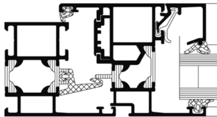
Schüco Window AWS 50 Scale 1:2
