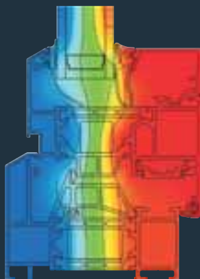
Schüco Fenster AWS 70 RL.HI Reduzierte Wärmeverluste Schüco window AWS 70 RL.HI Reduced heat loss
